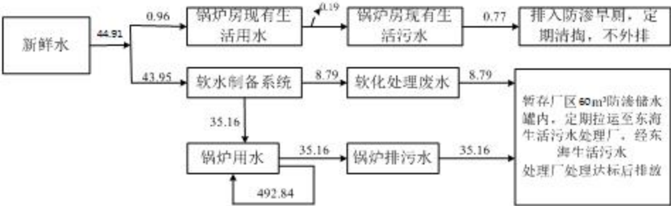
图 2-1 本项目建成后锅炉房供暖期水平衡图（单位：t/d）
