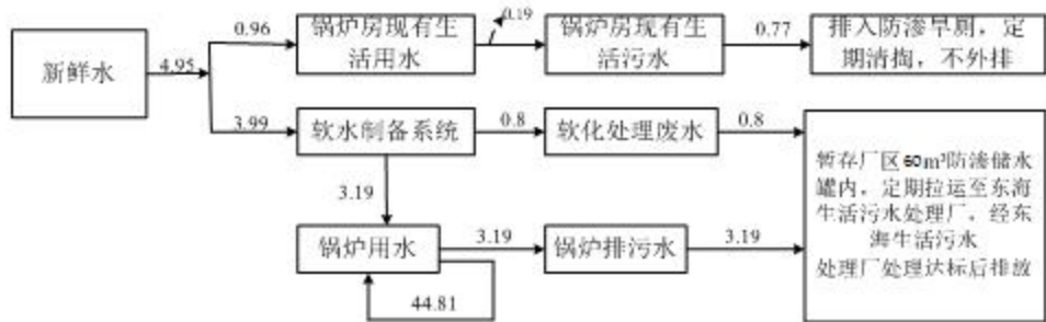
图 2-2 本项目非供暖期水平衡图（单位：t/d）
