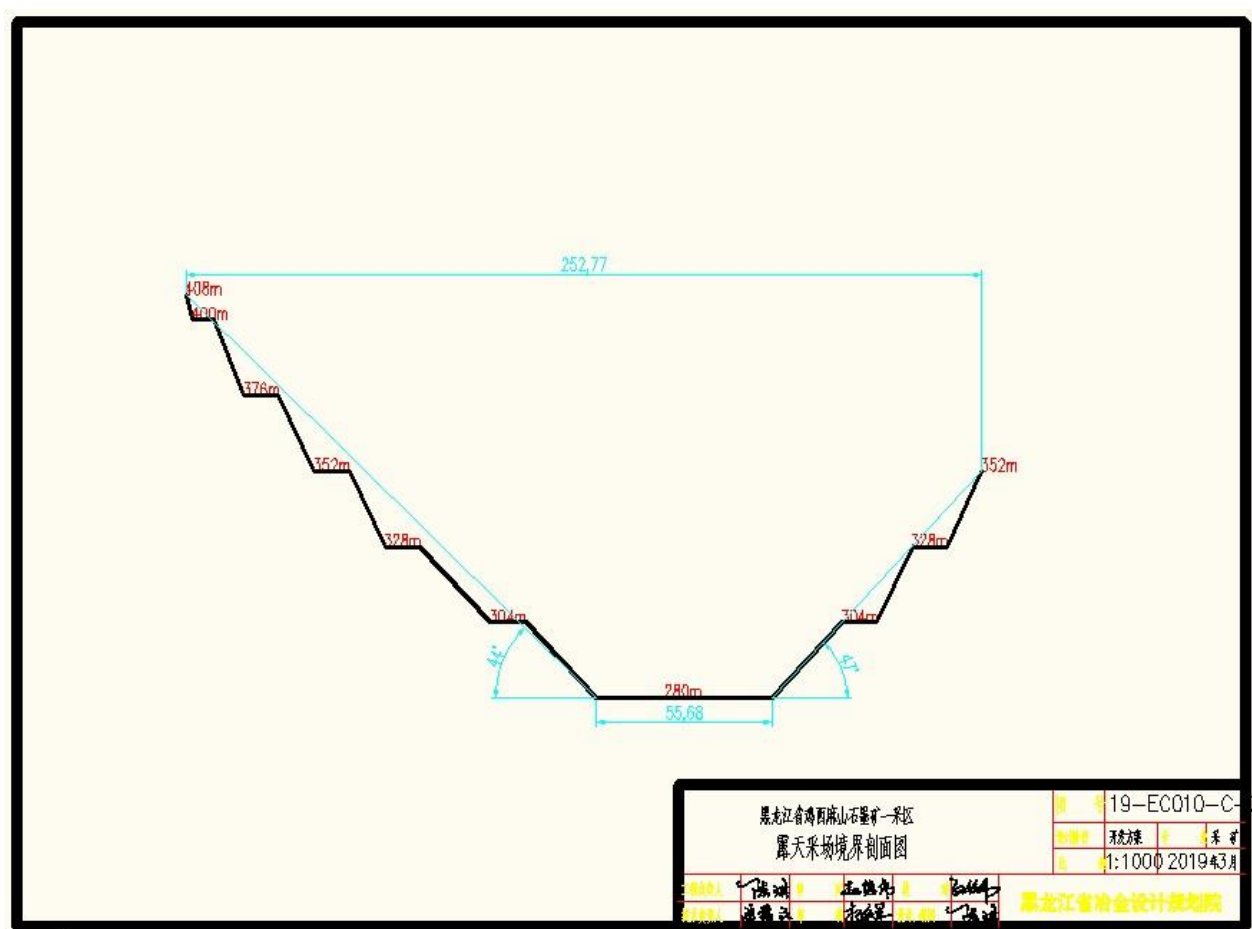
图 1-5 一区露天采场境界剖面图
