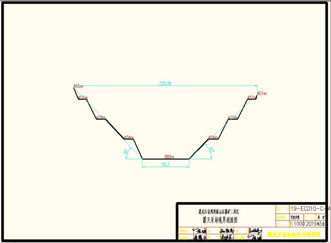
图 1-7 二区露天采场境界剖面图
