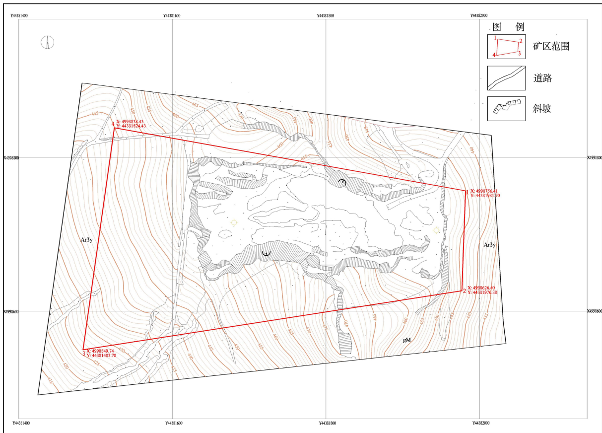
图 2-3 二区矿山地形地貌图
