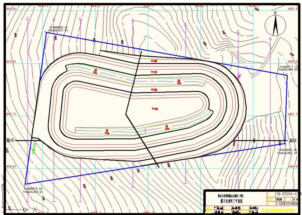
图 1-6 二区露天采场终了平面图
