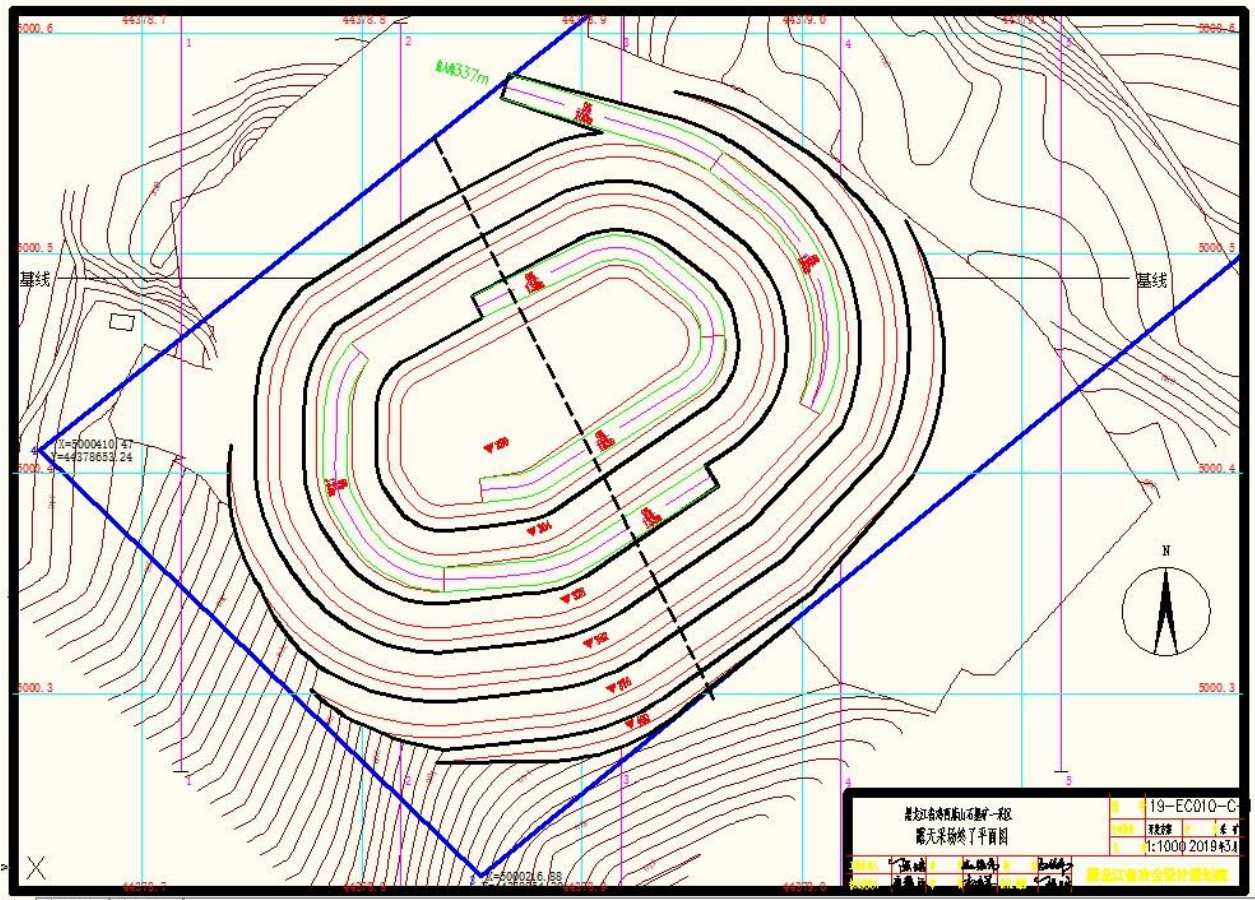
图 1-4 一区露天采场终了平面图
